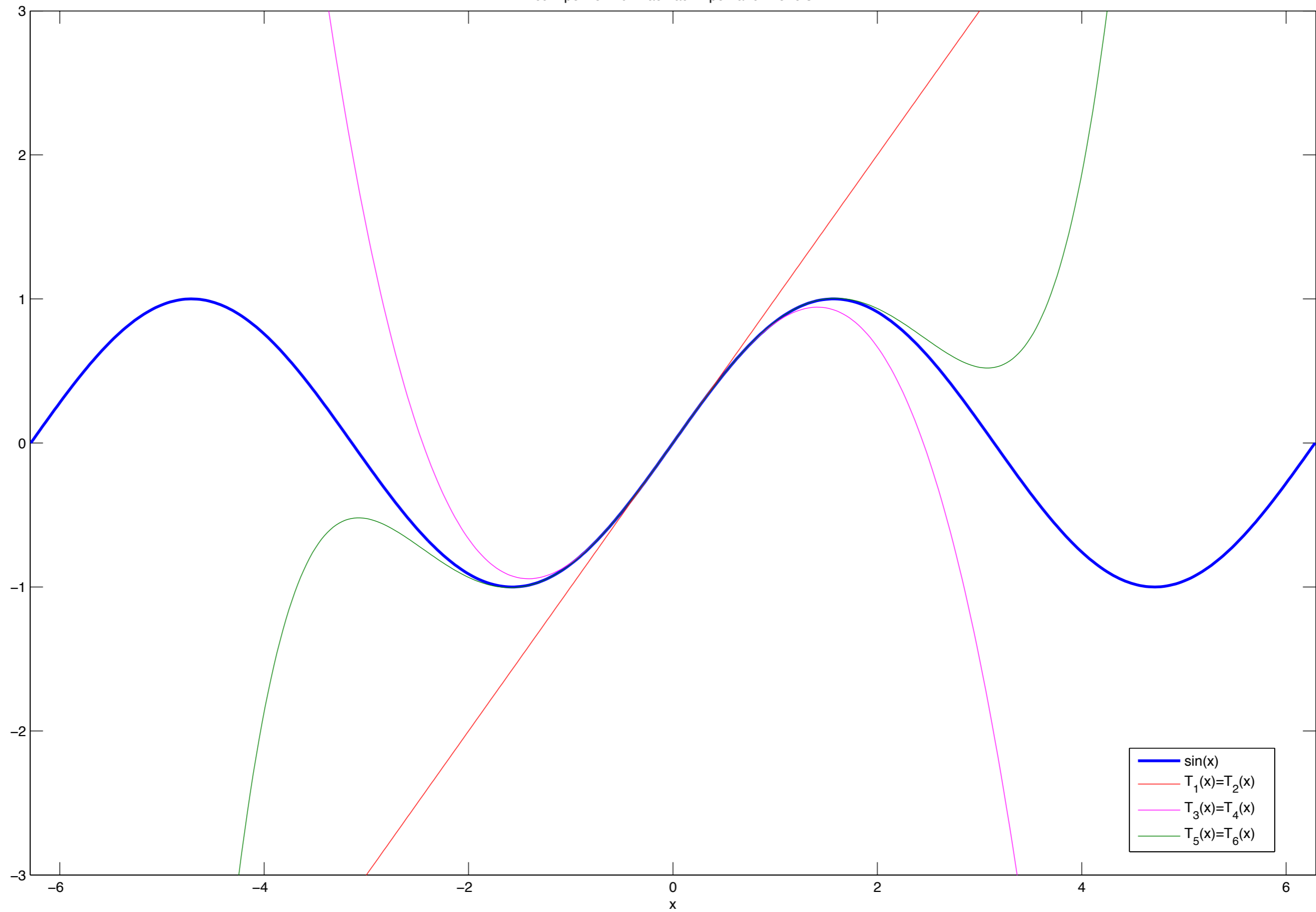
Alcuni polinomi di Mac Laurin per la funzione sin
